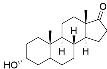
Androsterone 雄酮
