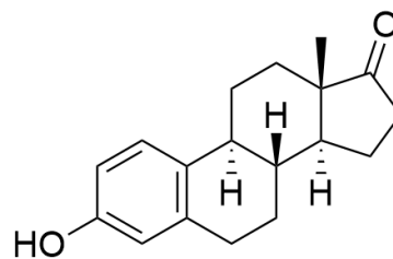
Estrone 雌酮
