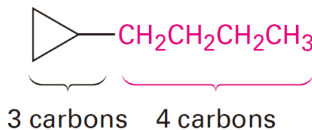
1-Cyclopropylbutane
