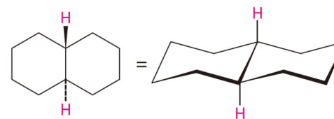
trans -Decalin
