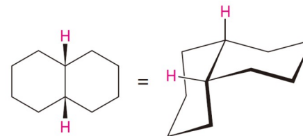
cis -Decalin
